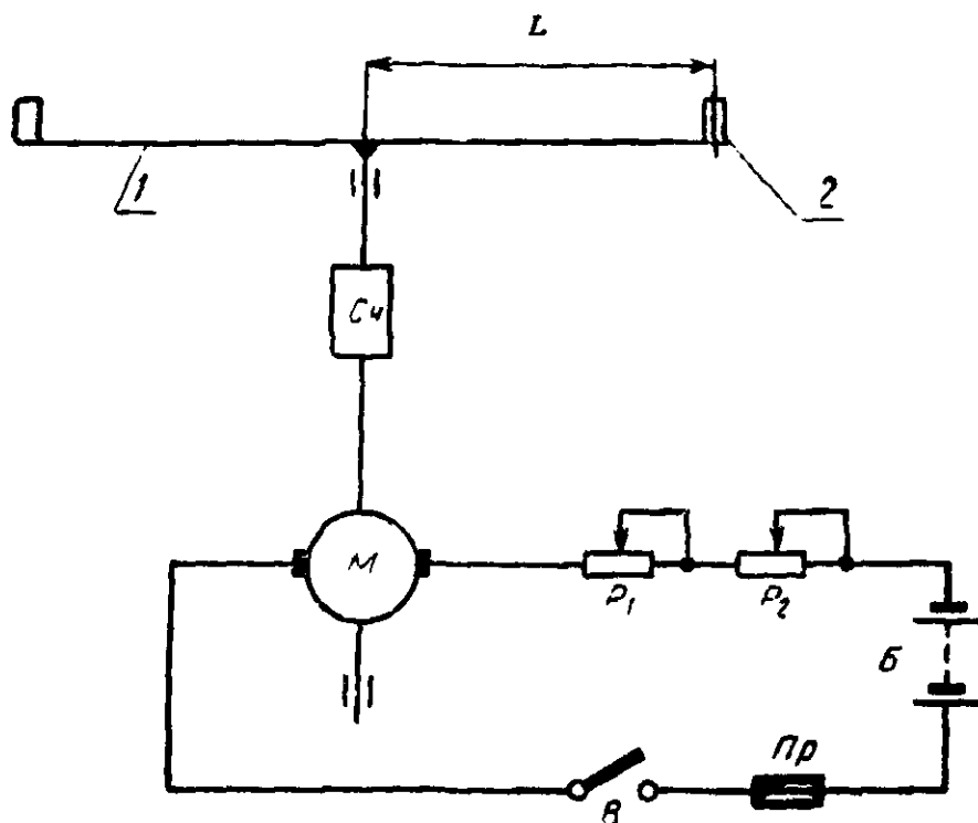
1—крестовина 2—стойка для крепления проверяемых анемометров, Cч—счетчик числа оборотов крестовины М—двигатель P 1 P 2 —реостаты Б—аккумуляторная батарея В—выключатель Пр предохранитель
