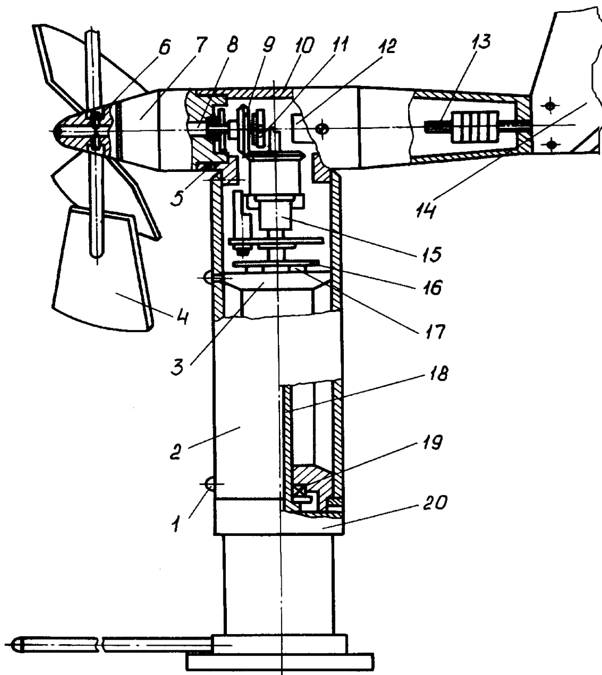
1, 6 – винты; 2, 18 – трубы; 3 – ступица; 4 – вертушка; 5 – стопорный винт; 7, 10 – корпуса; 8 – ось; 9 – шестерня; 11 – магнит; 12 – груз; 13 – шпилька; 14 – флюгарка; 15 – обойма; 16 – крышка; 17, 19 – подшипники; 20 – втулка.
